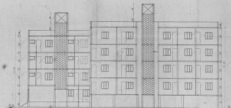
SECTION A-B
